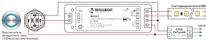
Рис. 2. Схема подключения диммера с использованием кнопки с подсветкой
