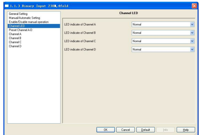
Fig.2.4 Parameter window "Channel LED"
