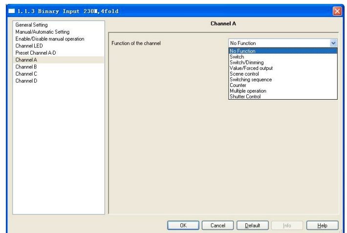
Fig.2.6 Parameter window "Channel X"
