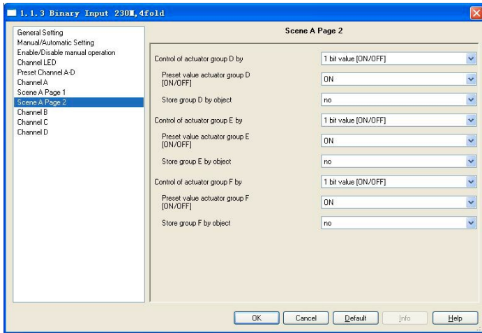
Fig.2.12 [2] Parameter window "Scene X Page 1/2, X"
