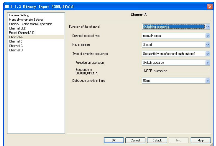
Fig.2.13 Parameter window "Switching sequence, X"
