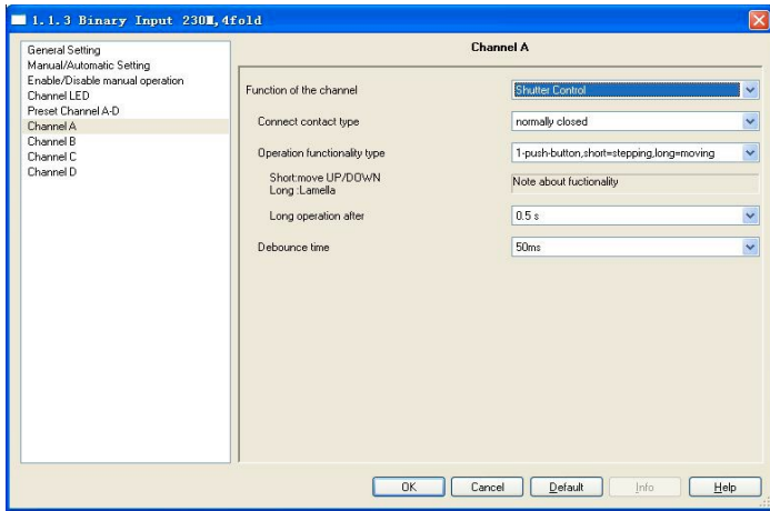
Fig.2.15 Parameter window "Shutter control, X"
