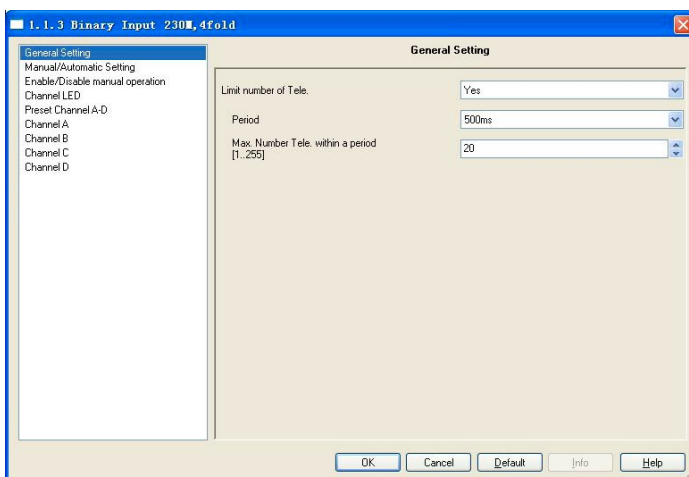
Fig.2.1 Parameter window "General Setting"
