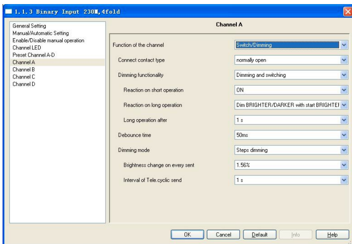
Fig.2.10 Parameter window “Switch / Dimming, X”
