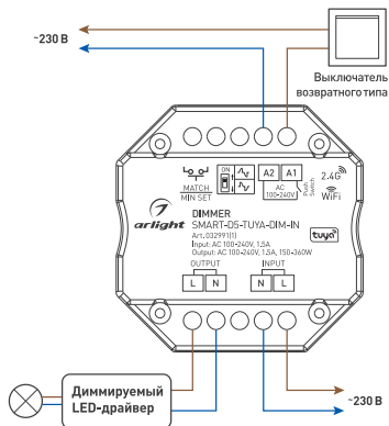
Рисунок 1. Схема подключения диммера SMART-D17-DIM
